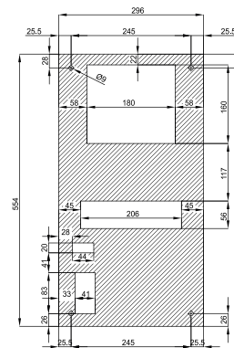
DIMA DI FORATURA CUTTING TEMPLATE
