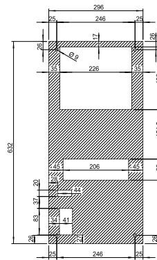
DIMA DI FORATURA CUTTING TEMPLATE
