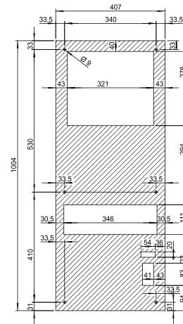
DIMA DI FORATURA CUTTING TEMPLATE
